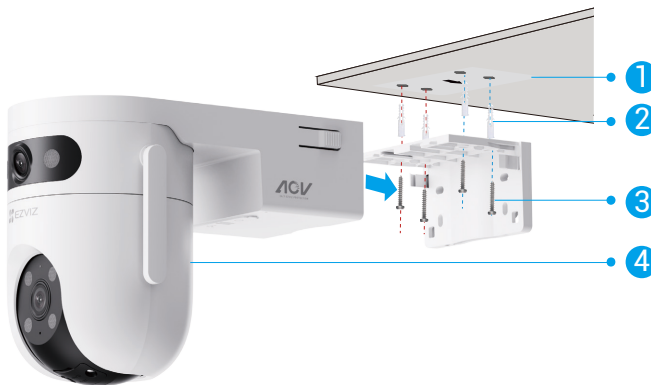
Fig. 1 Montering i loft
