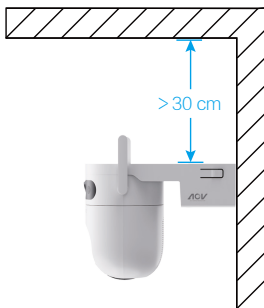
Fig. 2 Montering på væg
